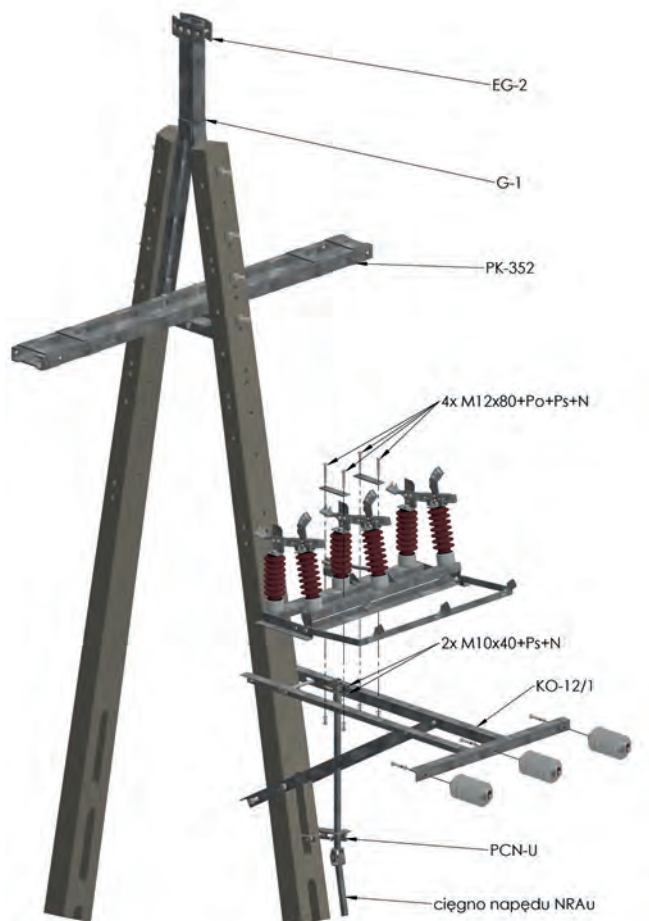
Rysunek montażowy
