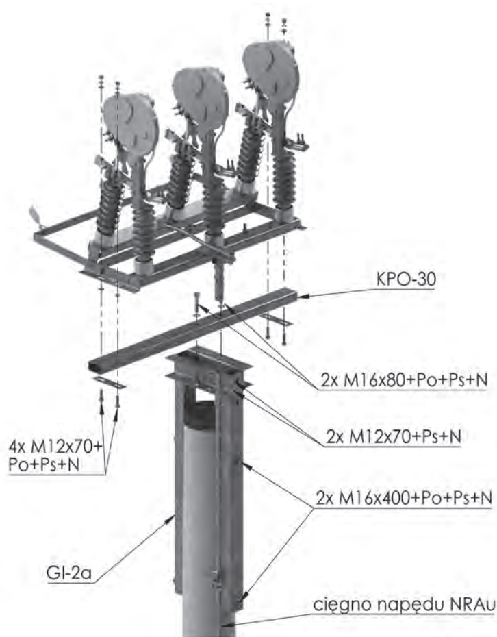
Rysunek montażowy
