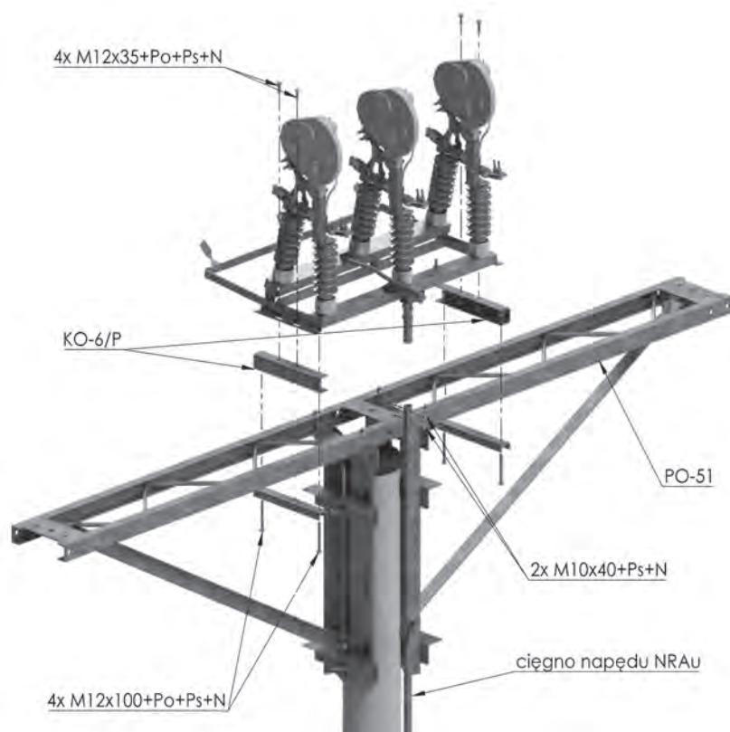
Rysunek montażowy
