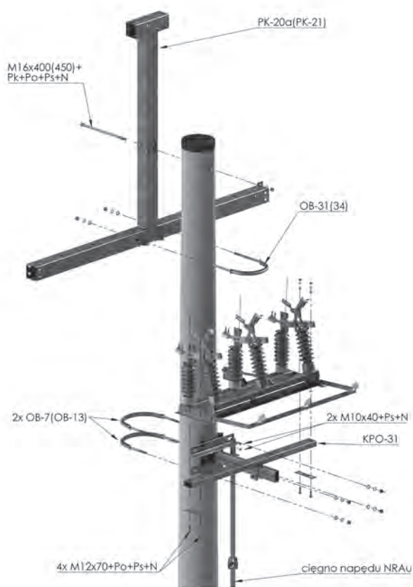
Rysunek montażowy
