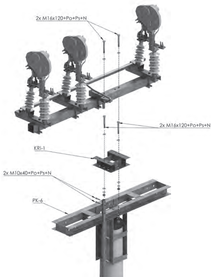
Rysunek montażowy
