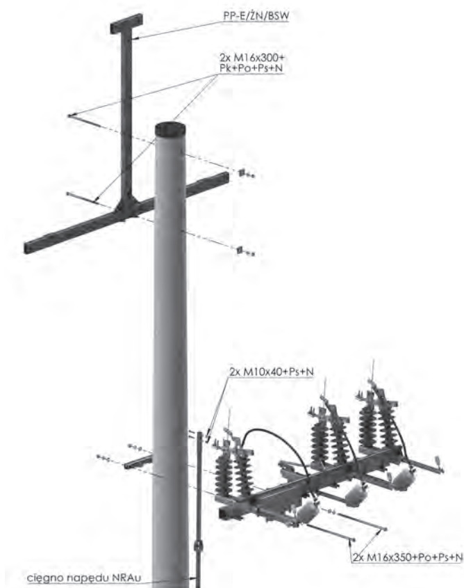
Rysunek montażowy
