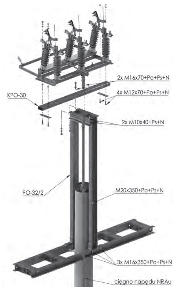
Rysunek montażowy
