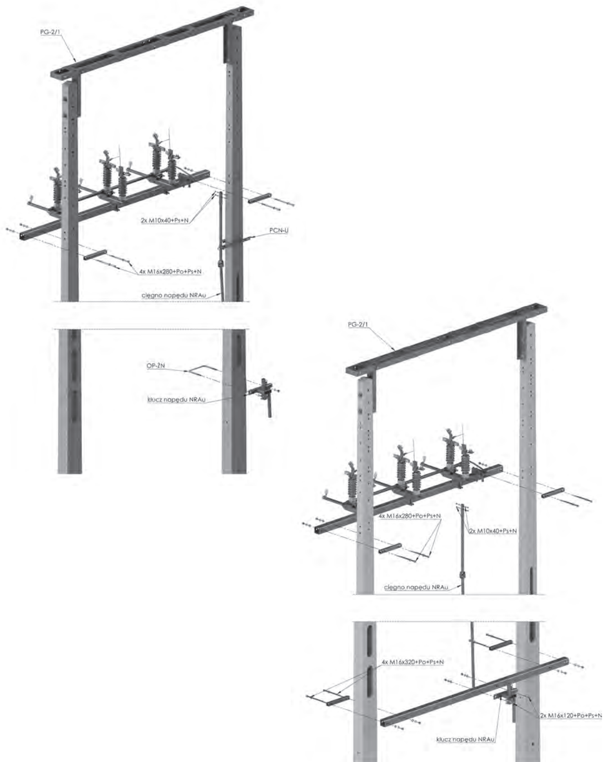
Rysunek montażowy
