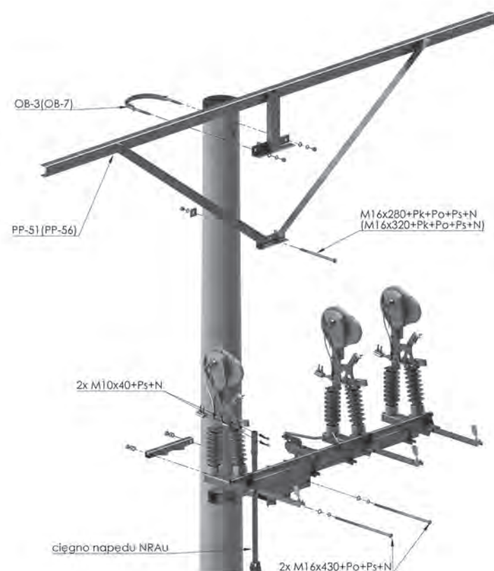
Rysunek montażowy
