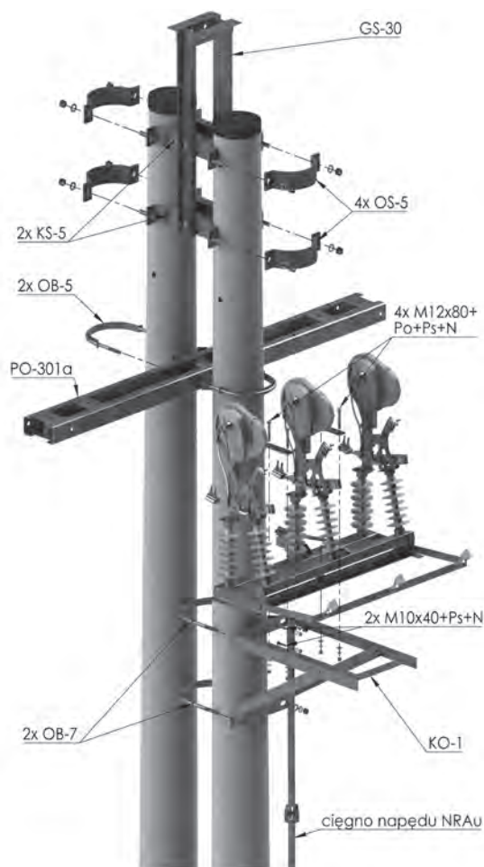
Rysunek montażowy
