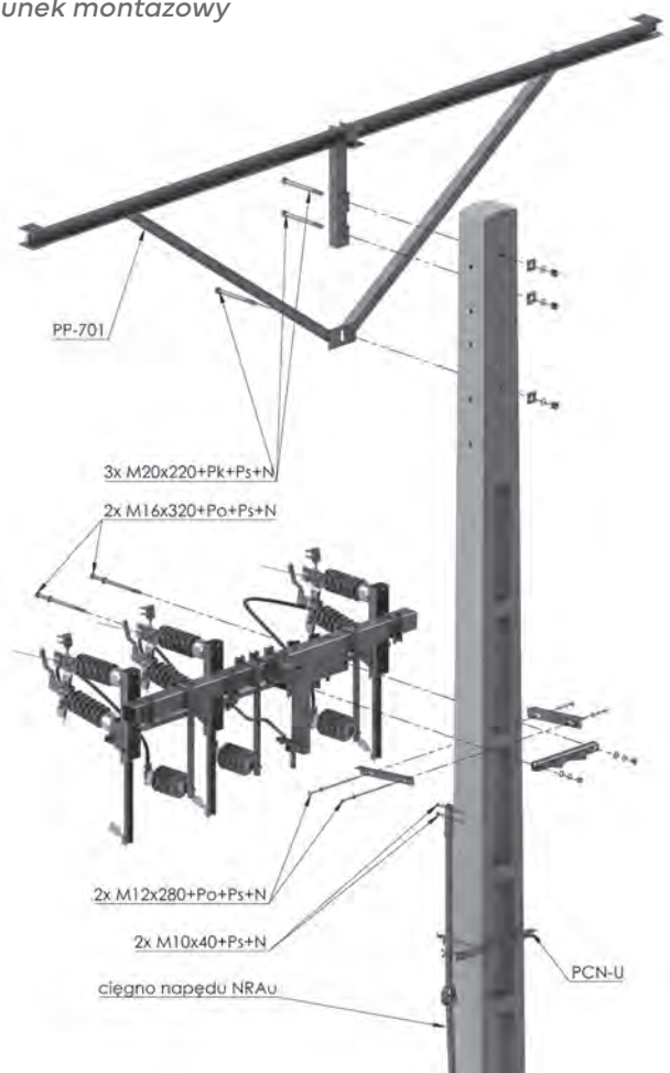
Rysunek montażowy
