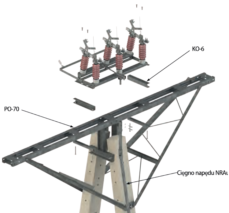
Rysunek montażowy
