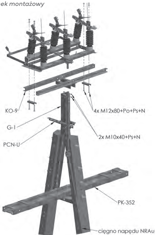
Rysunek montażowy
