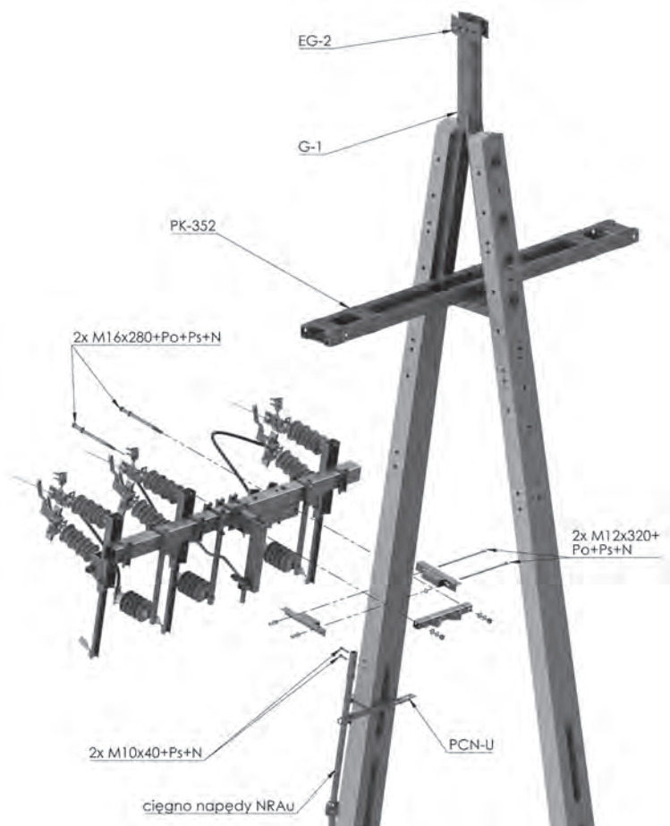
Rysunek montażowy
