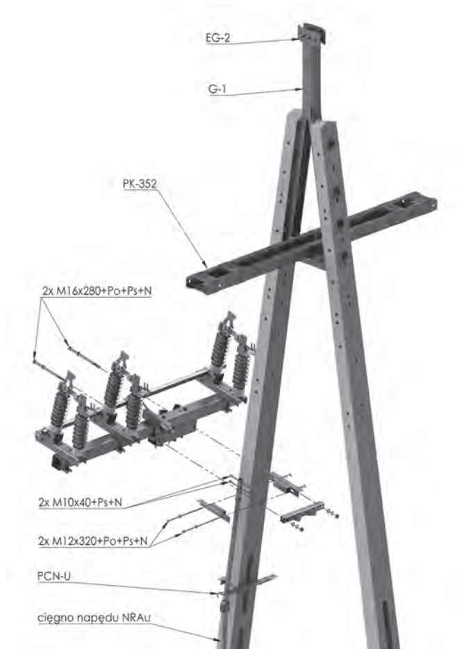
Rysunek montażowy
