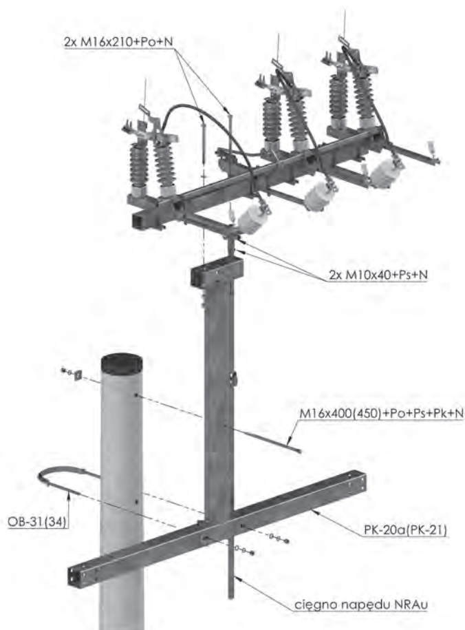
Rysunek montażowy
