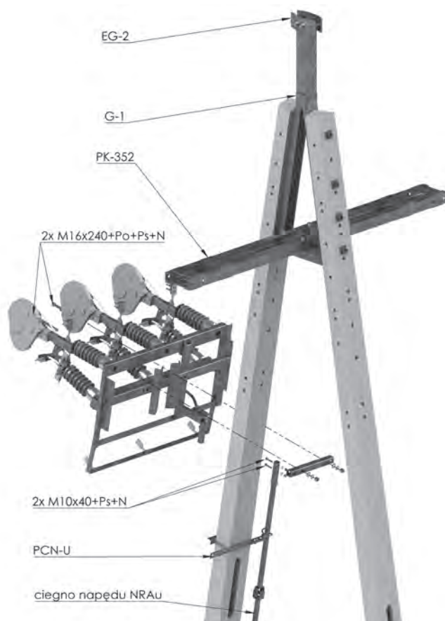
Rysunek montażowy
