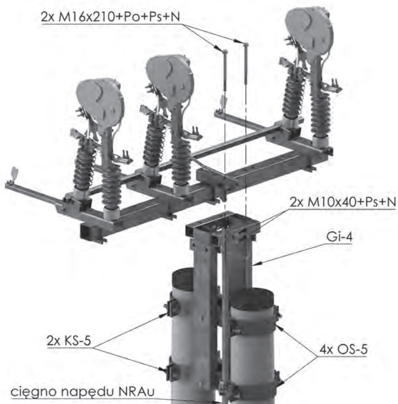
Rysunek montażowy
