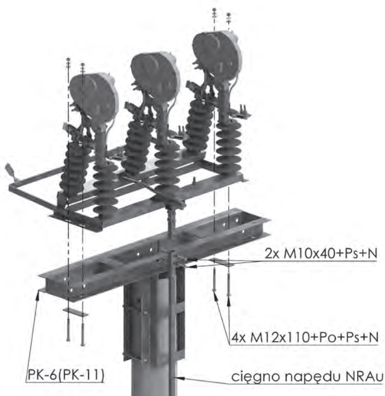
Rysunek montażowy
