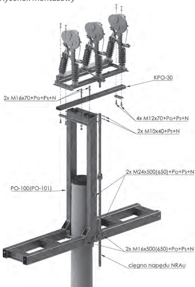
Rysunek montażowy
