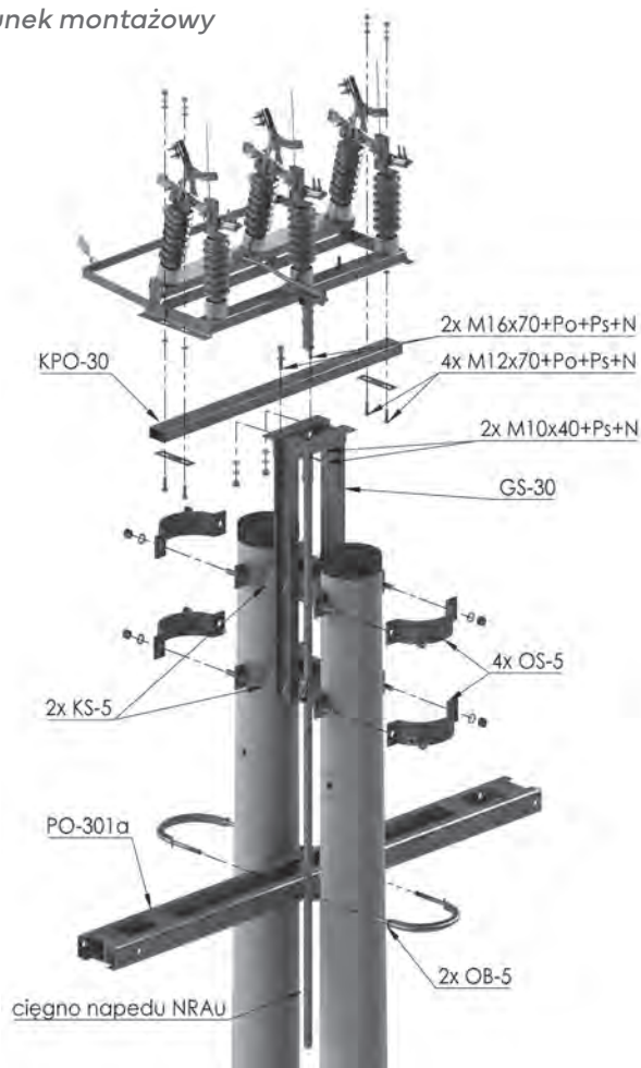
WIDOK A
