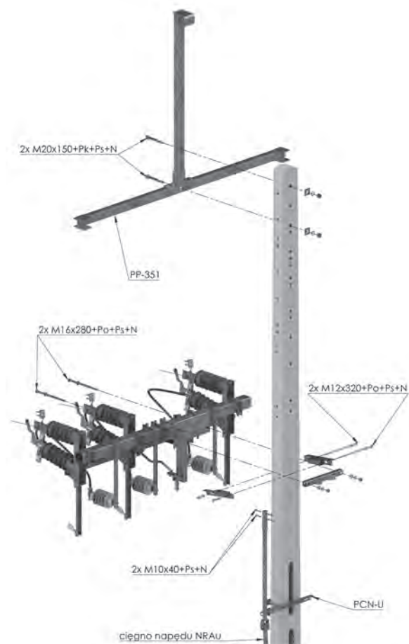
Rysunek montażowy
