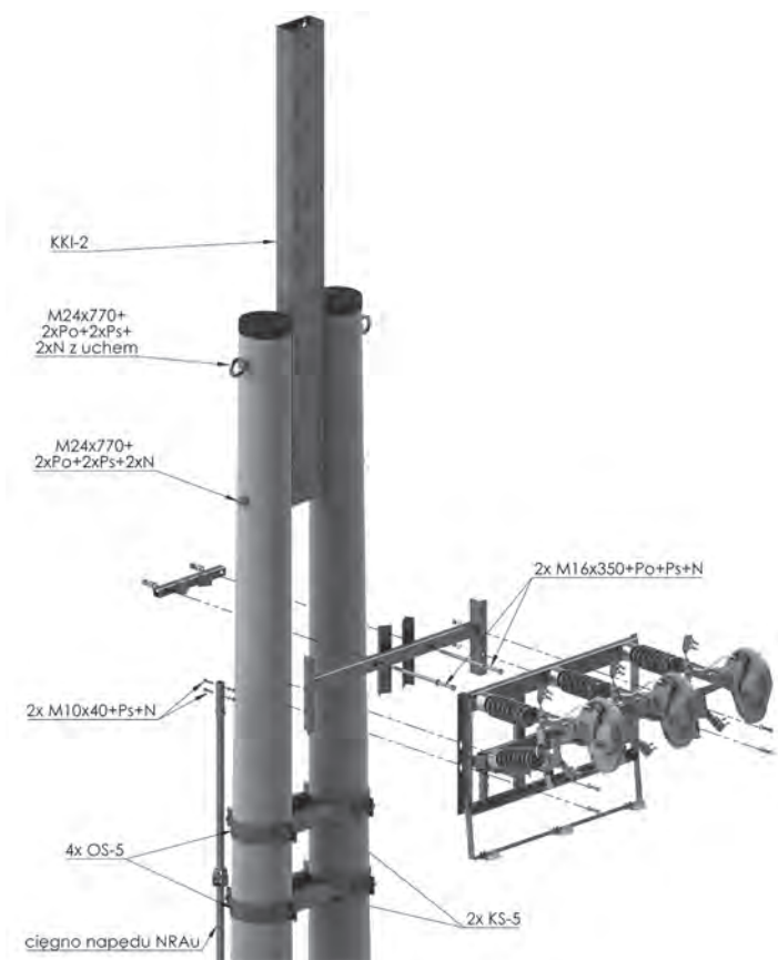
Rysunek montażowy
