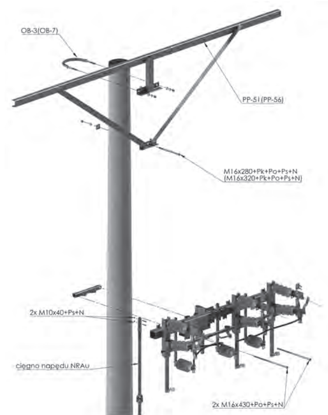
Rysunek montażowy
