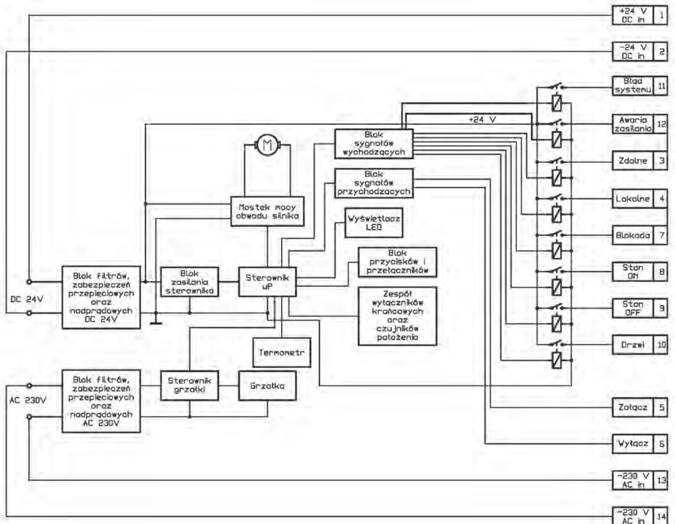
SCHEMAT BLOKOWY
