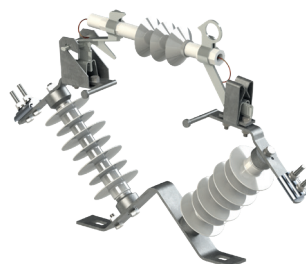
PBNVA-20/4S izolatory silikonowe
