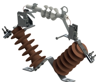
PBNVA-20/4K izolatory kompozytowe
