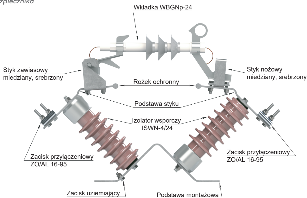
PBNVA-20/4 podstawa bezpiecznika
