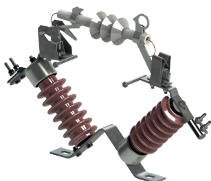
PBNVA-20/4 izolatory porcelanowe
