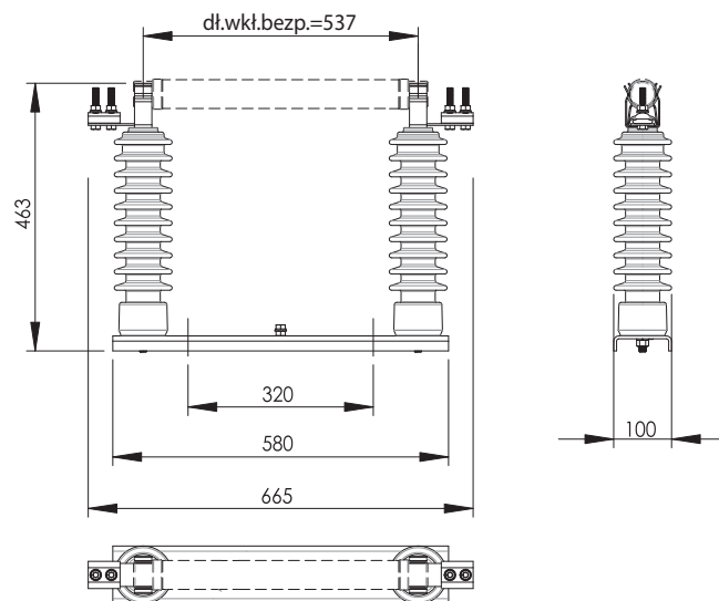
Podstawa bezpiecznikowa napowietrzna PBNWMA-30/50
