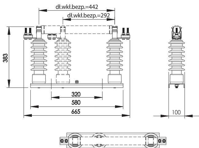
Podstawa bezpiecznikowa napowietrzna PBNWMA-24/50
